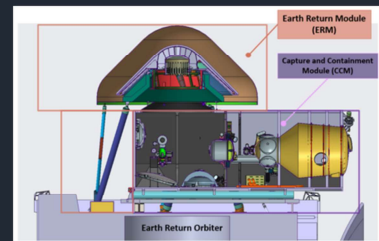
Earth Return Module (ERM)
